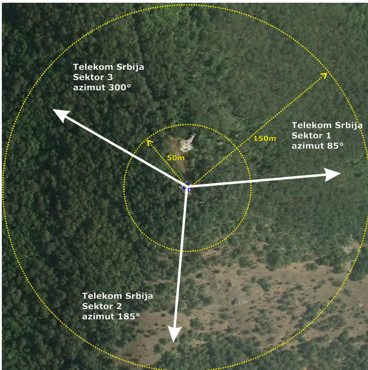
Slika 5.1 Dijagram zračenja radio bazne stanice „CA14 CAU14 CAL14 CAO14 Smedraž“
