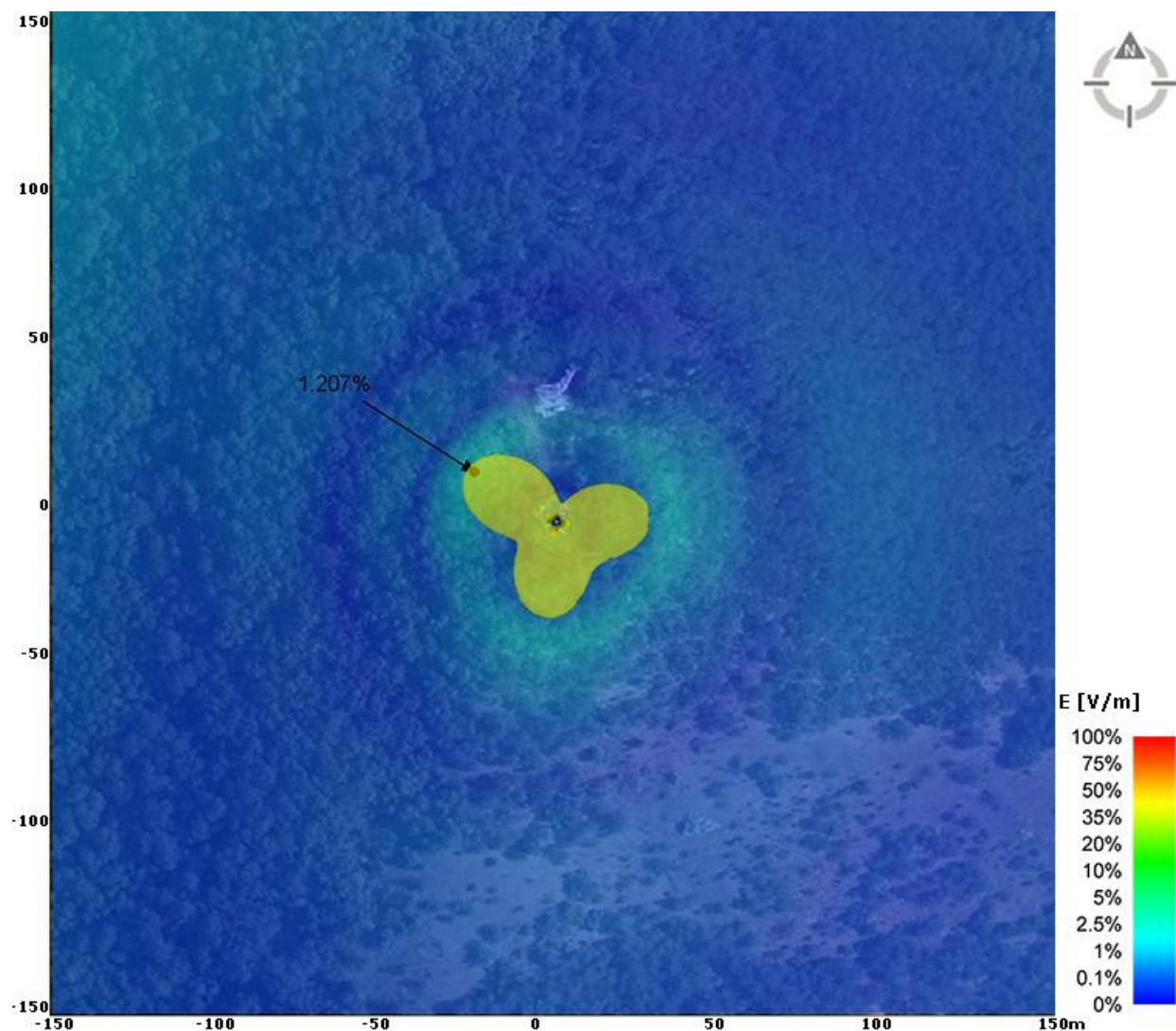
Slika 6.5.5 Rezultati proračuna- faktora izloženosti -u široj okolini na nivou tla, na visini +1,7m, za slučaj rada sistema- GSM900, UMTS2100, LTE1800 i LTE800 operatera- Telekom Srbija, za maksimalno opterećenje.
