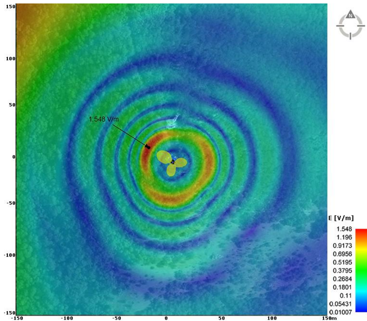
Slika 6.5.4 Rezultati proračuna jačine električnog polja u široj okolini na nivou tla, na visini +1,7m, za slučaj rada sistema LTE1800 operatera Telekom Srbija, za maksimalno opterećenje.
