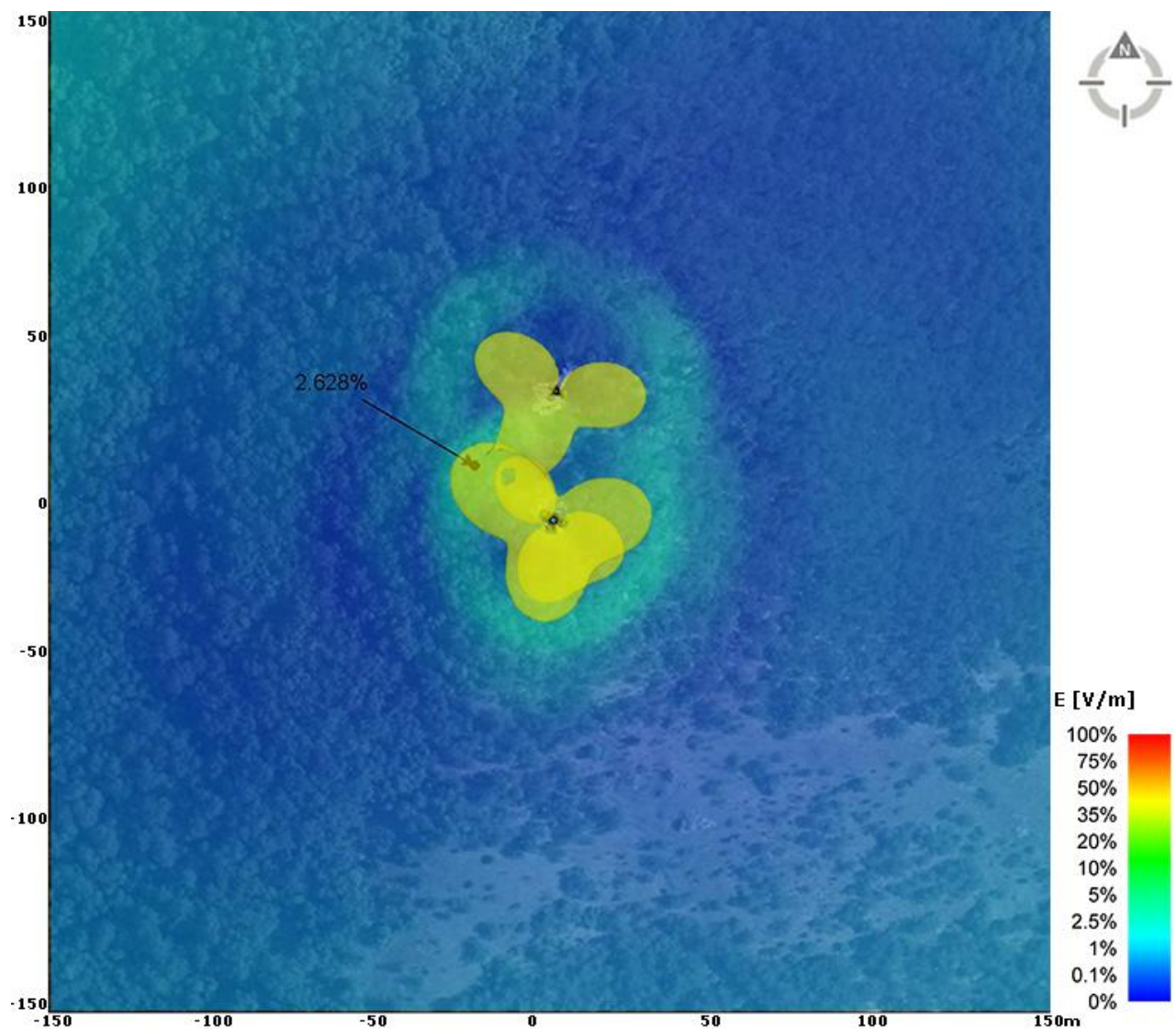
Slika 6.5.6 Rezultati proračuna faktora izloženosti u široj okolini na nivou tla, na visini +1,7m, za slučaj rada sistema GSM900, UMTS2100, LTE1800 i LTE800 operatera Telekom Srbija i postojeće opterećenje elektromagnetnom emisijom.
