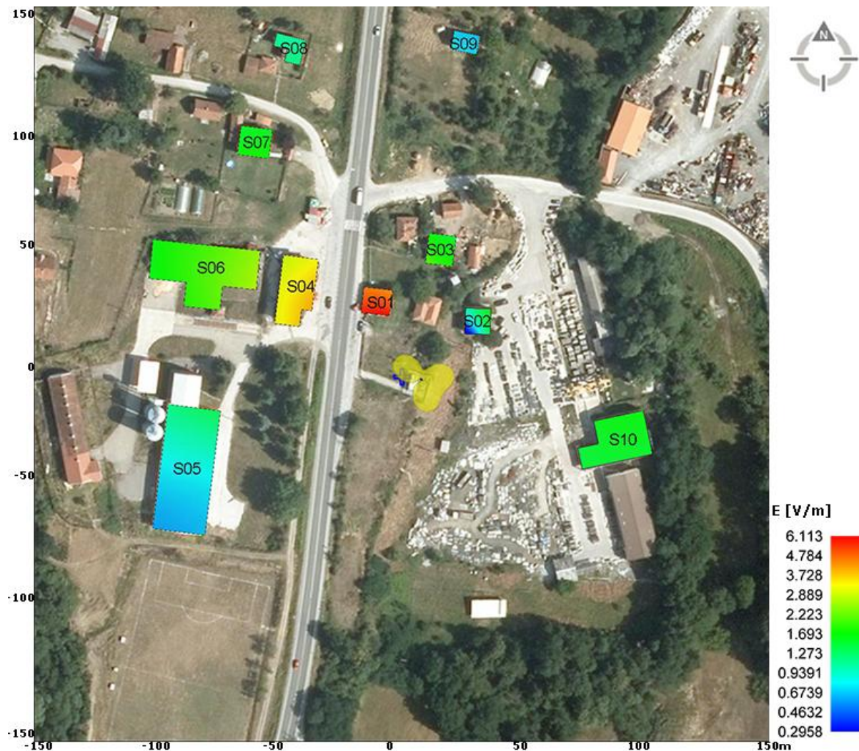
Slika 6.5.8 Rezultati proračuna jačine električnog polja u objektima na najizloženijim spratovima za slučaj rada sistema LTE800 operatera Telekom Srbija, za maksimalno opterećenje. Maksimum: 6.11 V/m.
