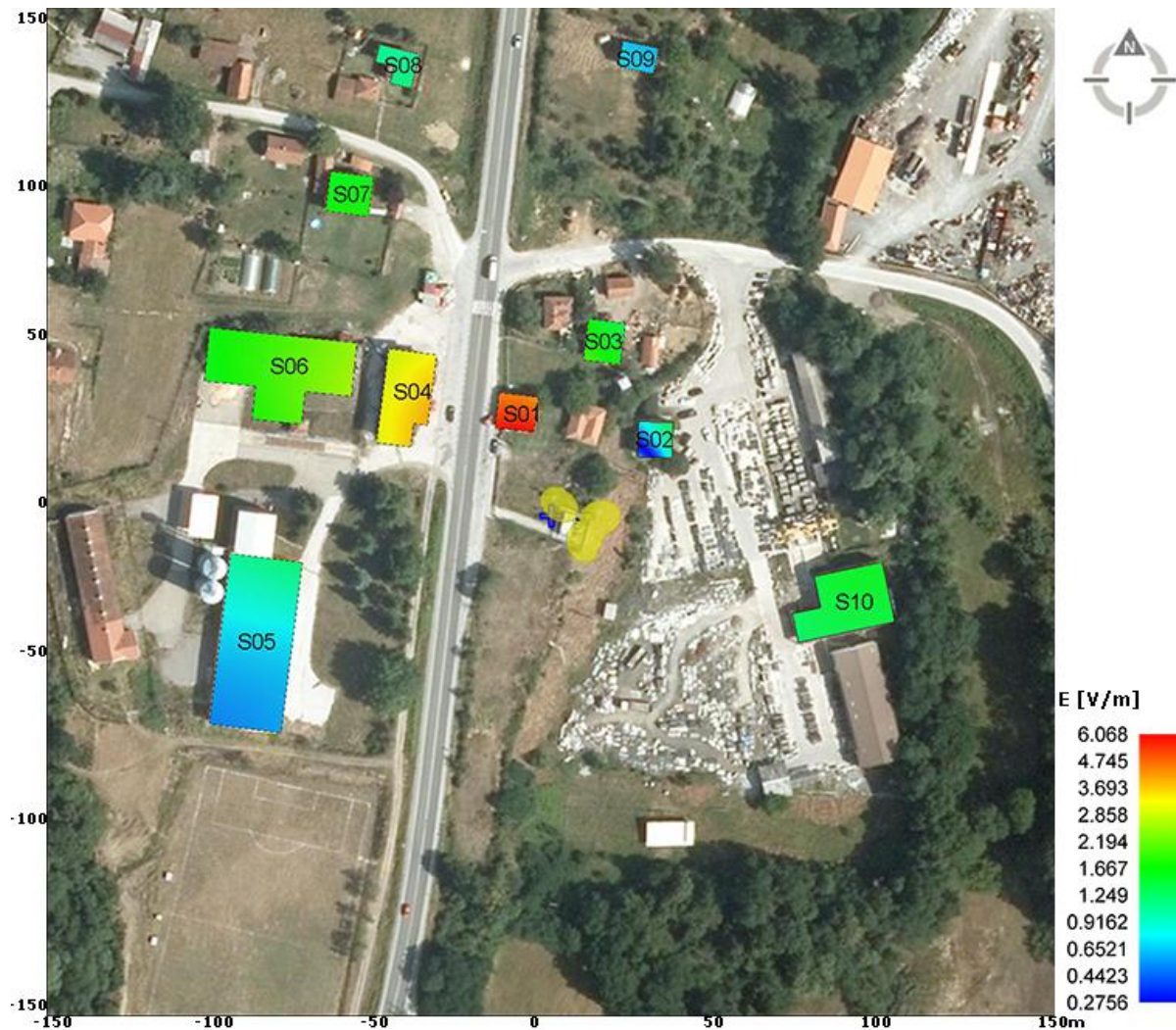
Slika 6.5.6 Rezultati proračuna jačine električnog polja u objektima na najizloženijim spratovima za slučaj rada sistema GSM900 operatera Telekom Srbija, za maksimalno opterećenje. Maksimum: 6.07 V/m.
