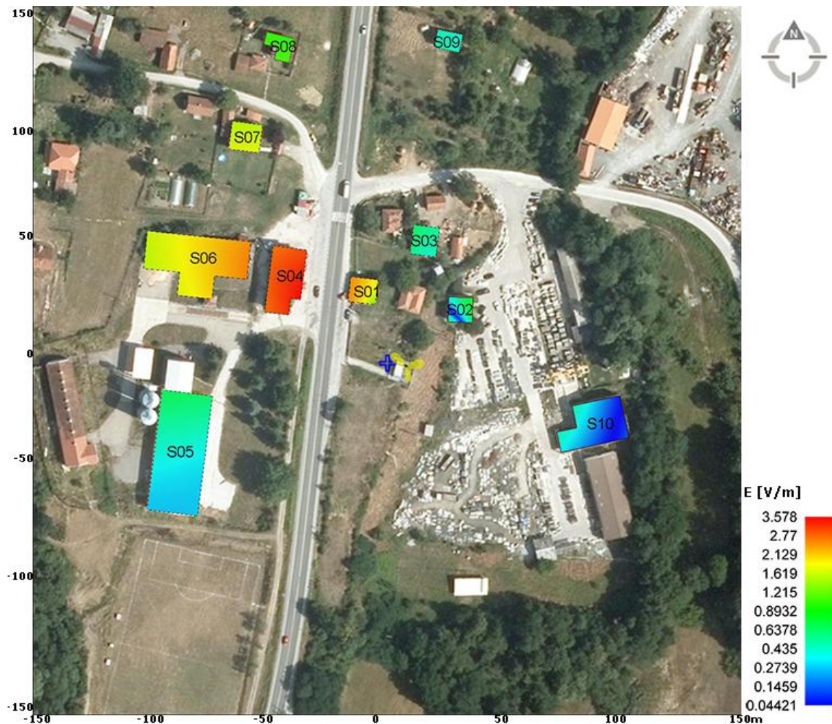
Slika 6.5.7 Rezultati proračuna jačine električnog polja u objektima na najizloženijim spratovima za slučaj rada sistema UMTS2100 operatera Telekom Srbija, za maksimalno opterećenje. Maksimum: 3.58 V/m.
