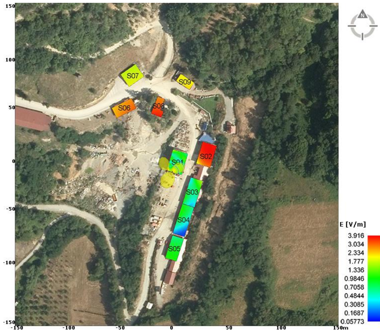
Slika 6.5.8 Rezultati proračuna jačine električnog polja u objektima na najizloženijim spratovima za slučaj rada sistema LTE800 operatera Telekom Srbija, za maksimalno opterećenje. Maksimum: 3.92 V/m.
