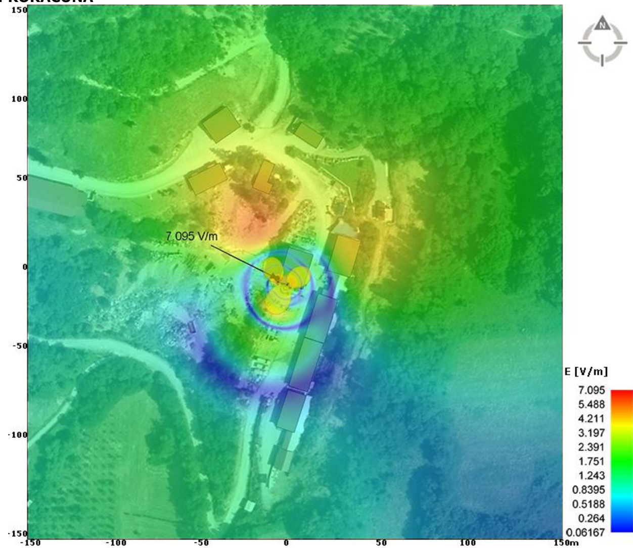
Slika 6.5.1 Rezultati proračuna jačine električnog polja u široj okolini na nivou tla, na visini +1,7m, za slučaj rada sistema GSM900 operatera Telekom Srbija, za maksimalno opterećenje.
