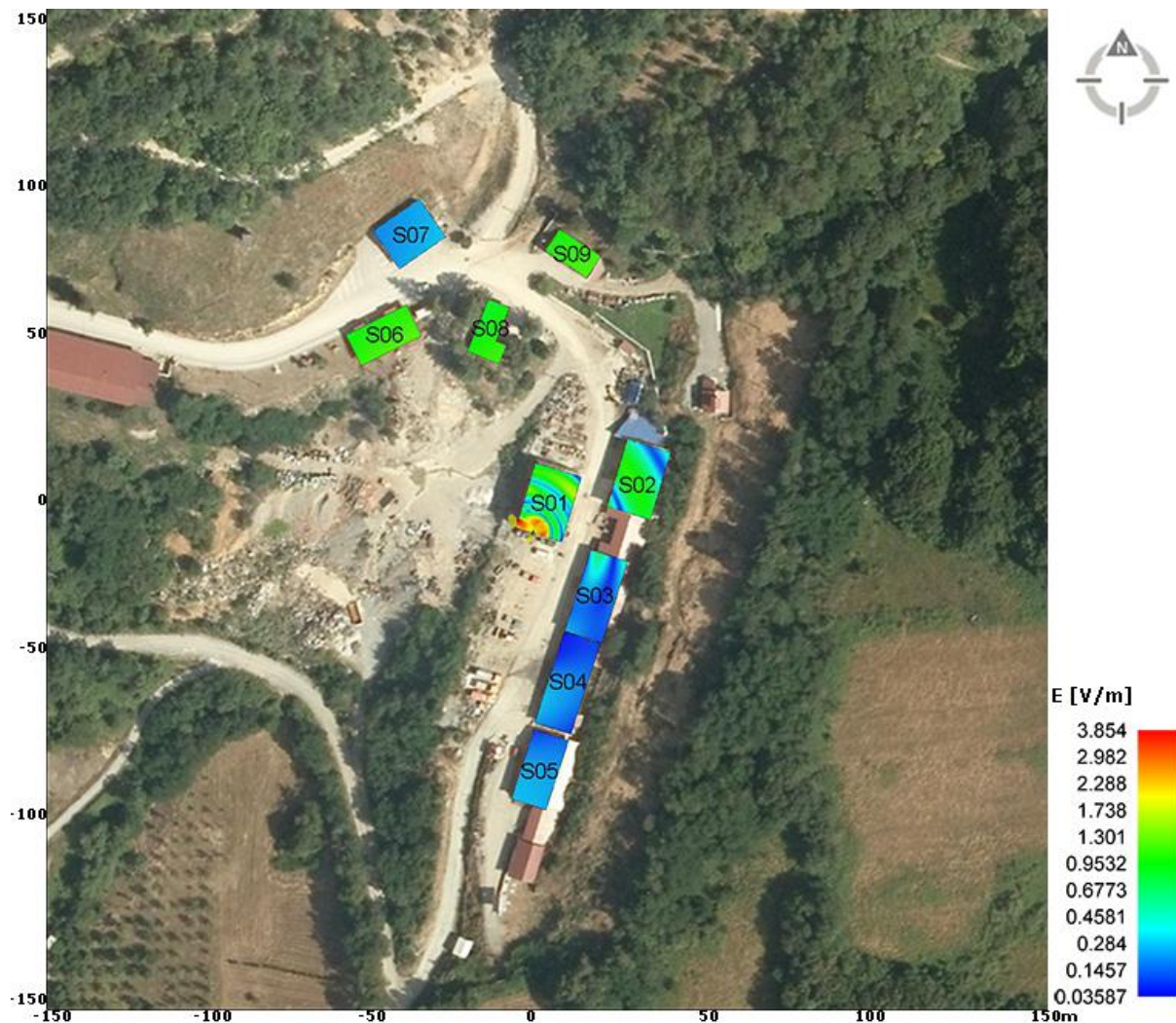
Slika 6.5.7 Rezultati proračuna jačine električnog polja u objektima na najizloženijim spratovima za slučaj rada sistema UMTS2100 operatera Telekom Srbija, za maksimalno opterećenje. Maksimum: 3.85 V/m.
