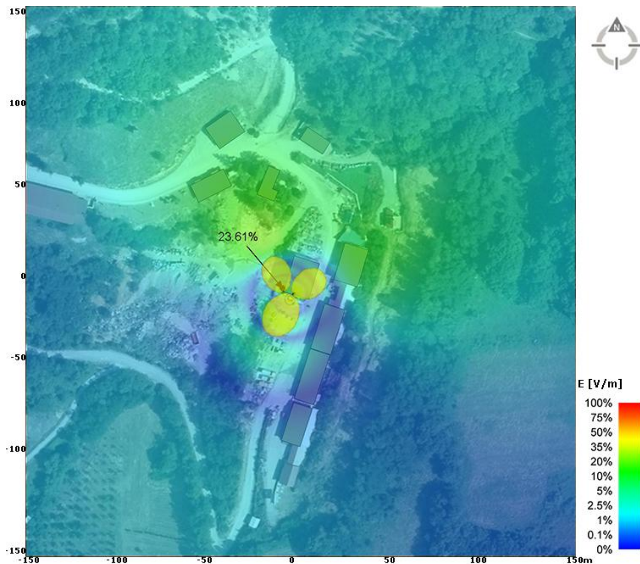
Slika 6.5.4 Rezultati proračuna faktora izloženosti u široj okolini na nivou tla, na visini +1,7m, zaslučaj rada sistema GSM900, UMTS2100 i LTE800 operatera Telekom Srbija, za maksimalno opterećenje.
