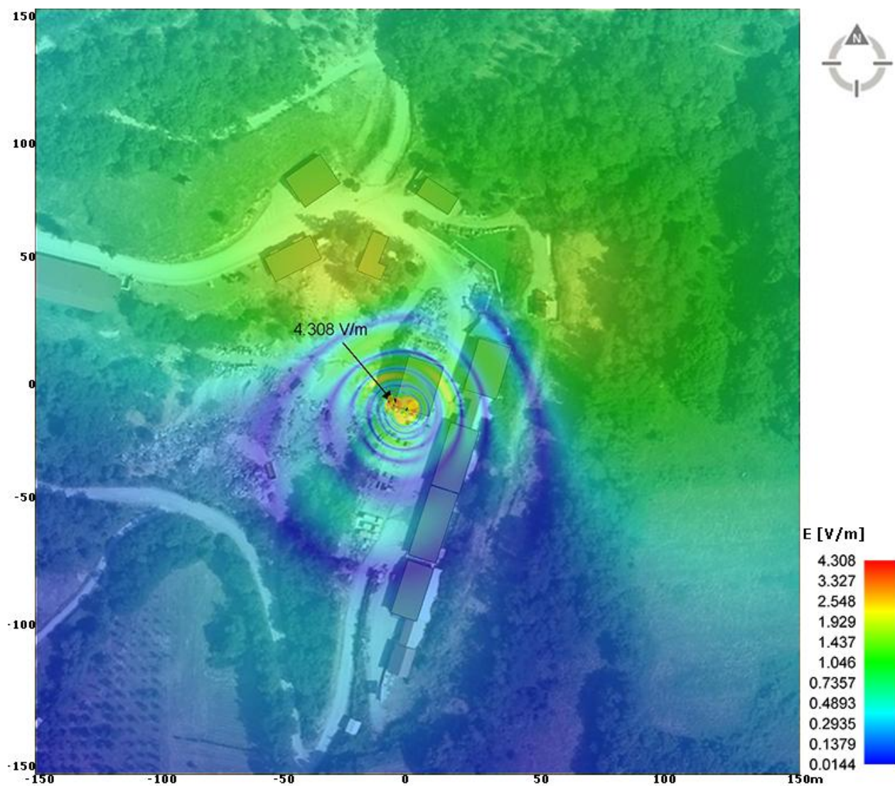
Slika 6.5.2 Rezultati proračuna jačine električnog polja u široj okolini na nivou tla, na visini +1,7m, za slučaj rada sistema UMTS2100 operatera Telekom Srbija, za maksimalno opterećenje.
