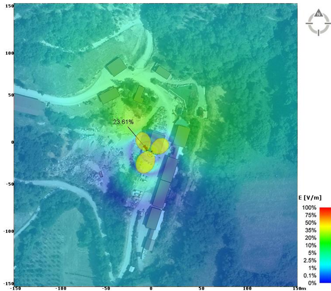
Slika 6.5.5 Rezultati proračuna faktora izloženosti u široj okolini na nivou tla, na visini +1,7m, zaslužaj rada sistema GSM900, UMTS2100 i LTE800 operatera Telekom Srbija i postojeće opterećenje elektromagnetnom emisijom.
