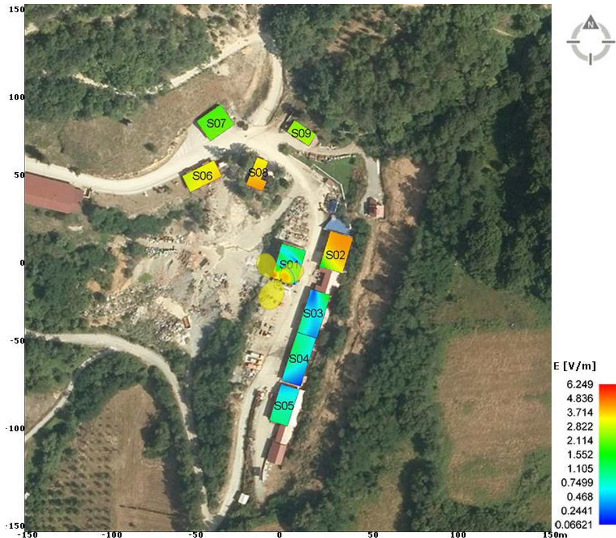
Slika 6.5.6 Rezultati proračuna jačine električnog polja u objektima na najizloženijim spratovima za slučaj rada sistema GSM900 operatera Telekom Srbija, za maksimalno opterećenje. Maksimum: 6.25 V/m.
