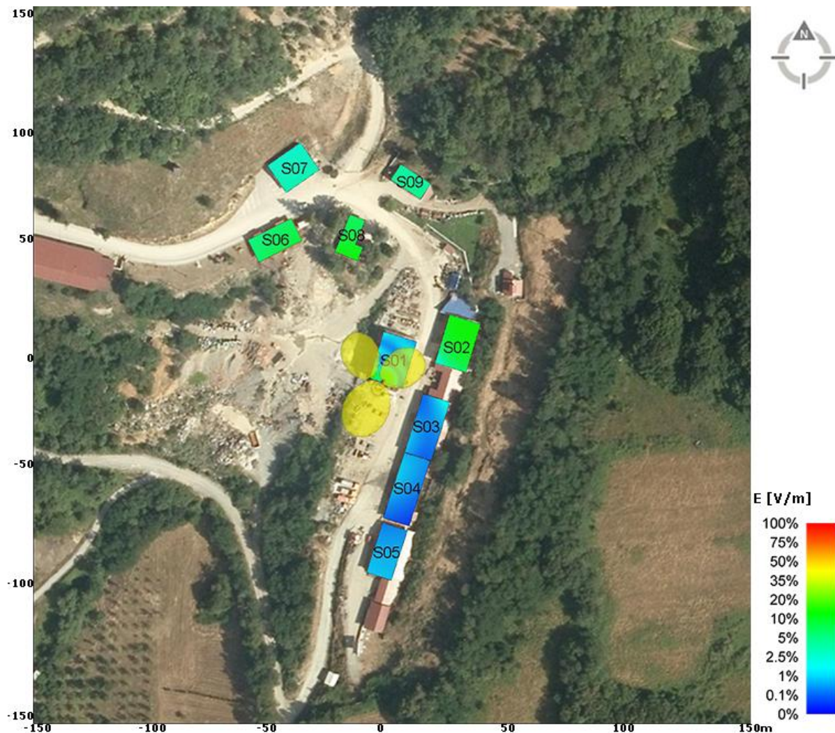
Slika 6.5.10 Rezultati proračuna faktora izloženosti u objektima na najizloženijim spratovima, za slučaj rada sistema UMTS2100, GSM900 i LTE800 operatera Telekom Srbija i postojeće opterećenje elektromagnetnom emisijom
