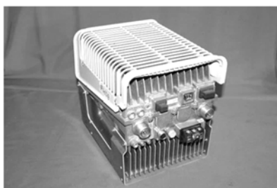
Slika 3.7 Izgled jednosektorskih Nokia Flexi radio modula
