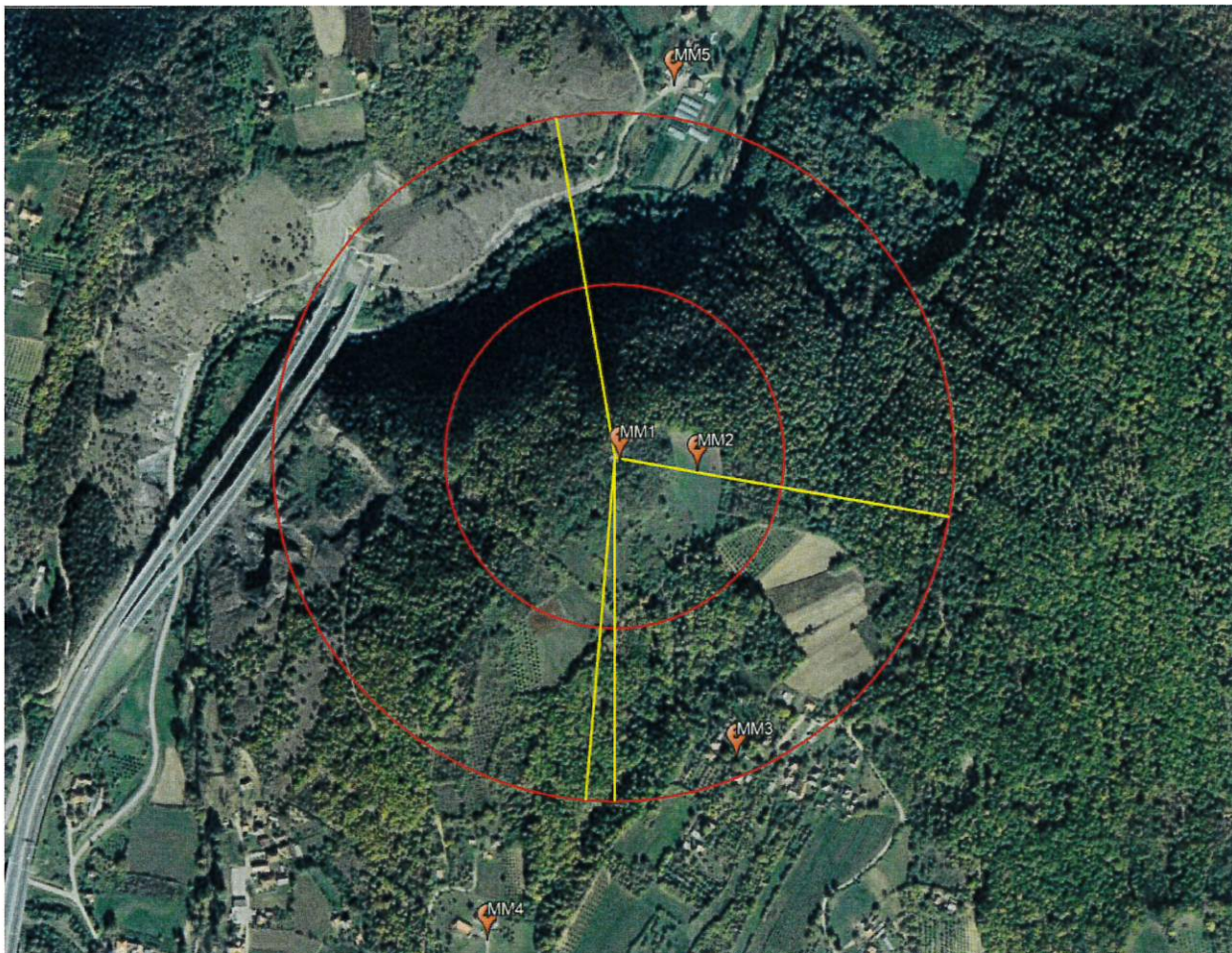
Slika 8: Prikaz Mernih Mesta u lokalnoj zoni BS Telekom Srbija Brđani (Koridor 10)
