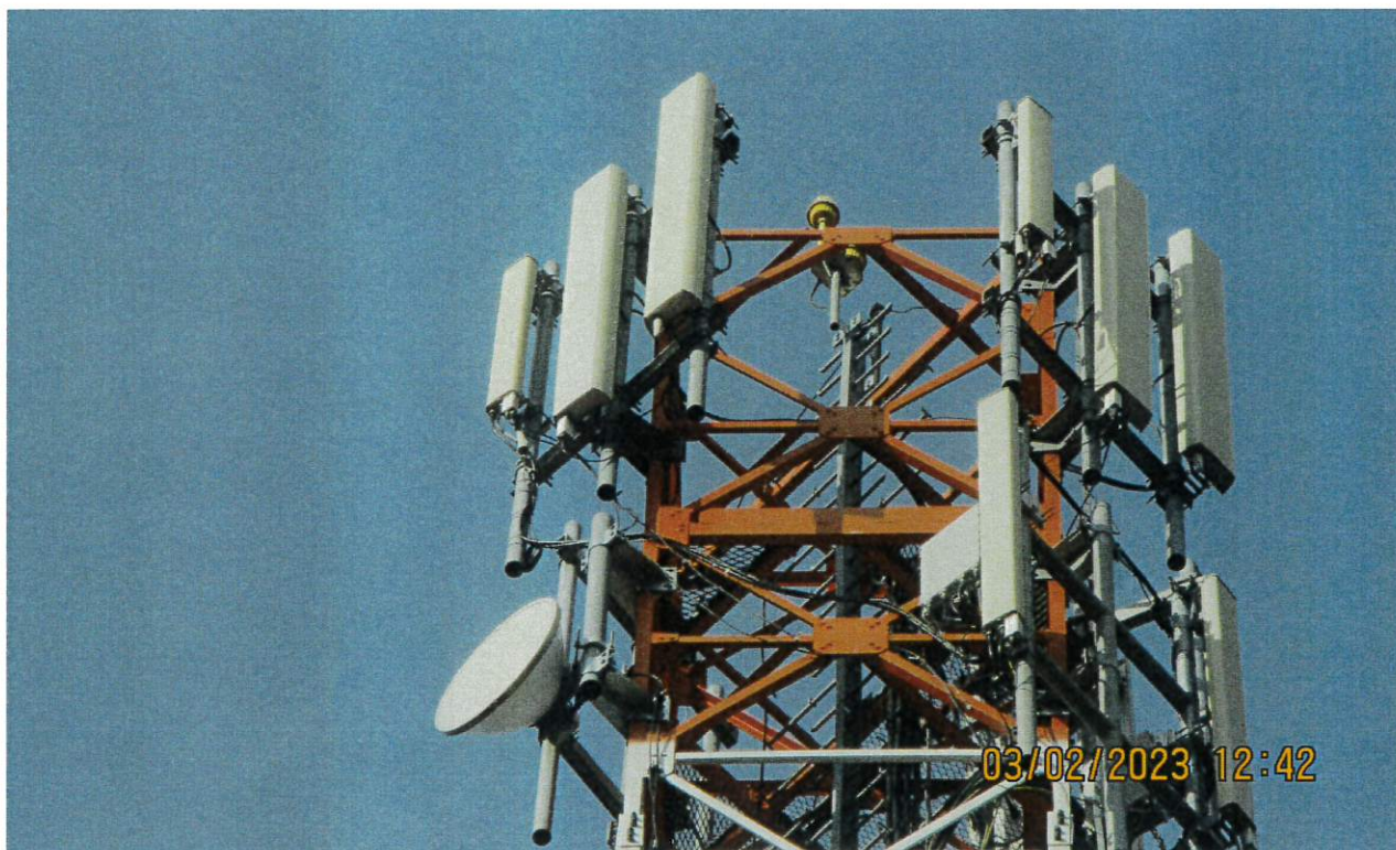
Slika 4 : Prikaz antena sektora 1 i 2 BS Brđani (Koridor 10) operatora Telekom Srbija
