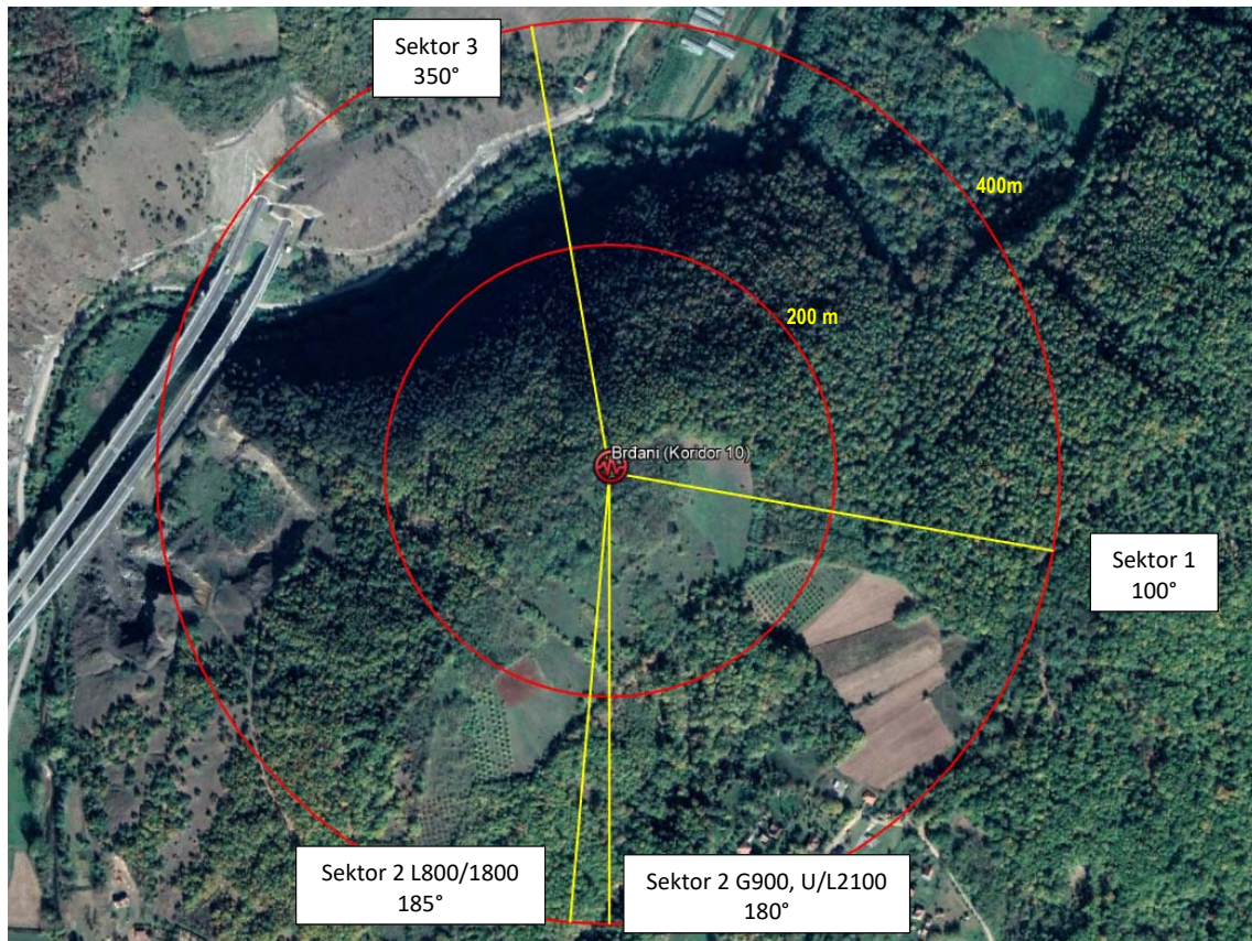
Slika 5.5 Pravci zračenja antenskog sistema BS BRĐANI (KORIDOR10) – CA83/CAU83/CAL83/CAO83/CAJ83
