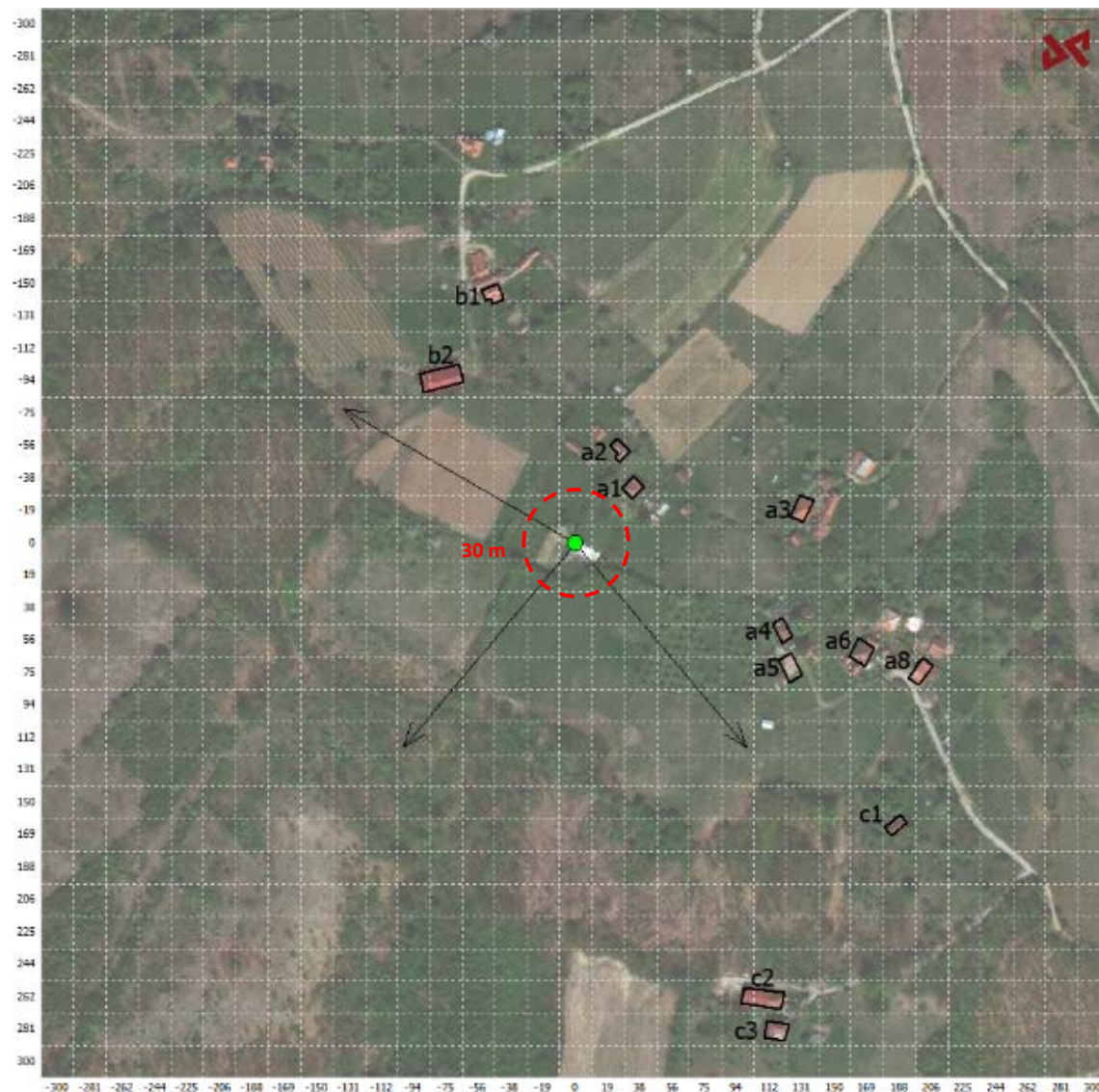
Slika 2.4 Prikaz pravaca zračenja antena i pozicije okolnih objekata
