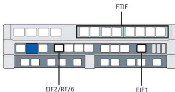
Slika 3.6 Transportni interfejsi FSMF modula
