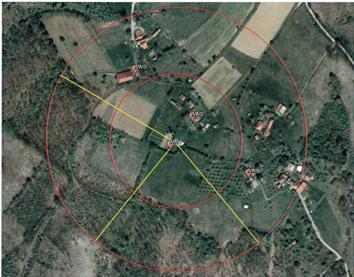
Slika 8: Prikaz Mernih Mesta u lokalnoj zoni BS Telekom Srbija Boljkovci
