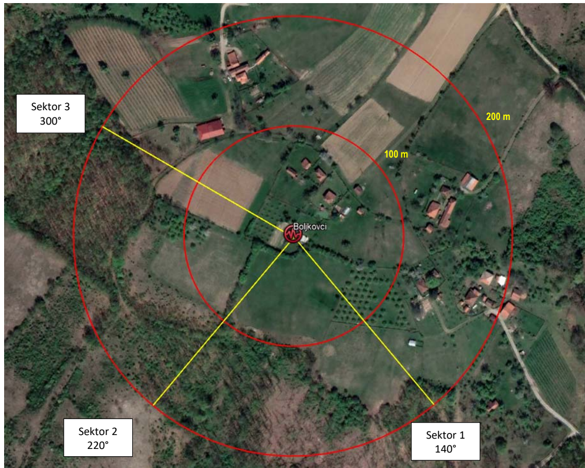
Slika 5.5 Pravci zračenja antenskog sistema BS BOLJKOVCI – CA84/CAU84/CAL84/CAO84/CAJ84
