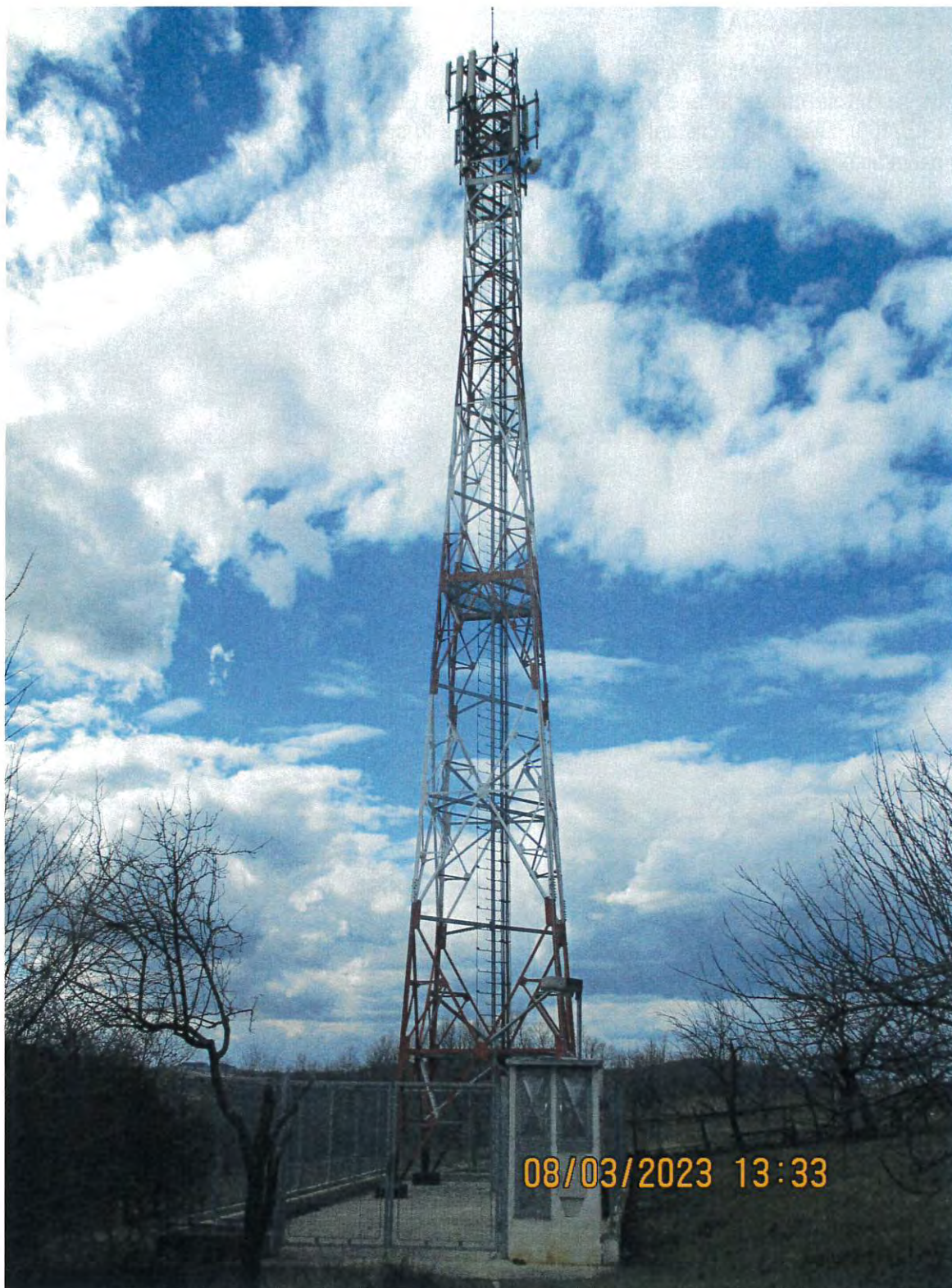
Slika 3: Prikaz antenskog stuba na kom se nalazi antenski sistem bazne stanice Boljkovci, operatora Telekom Srbija
